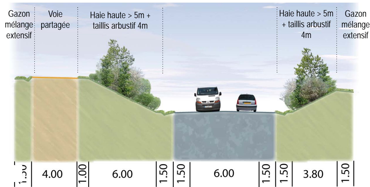
COUPE E - F
