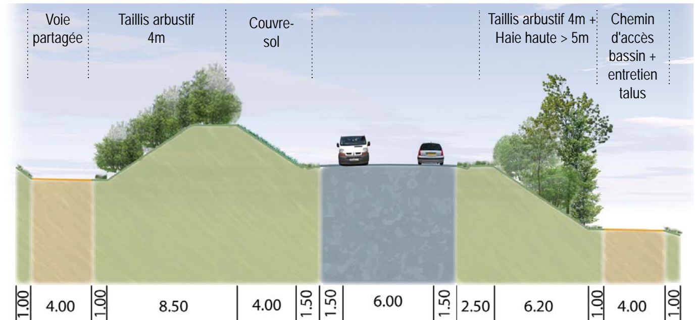
COUPE C-D PERCEPTION DE L'AUTOMOBILISTE UNE AMBIANCE INTIME BOCAGERE Profils 22 à 34
