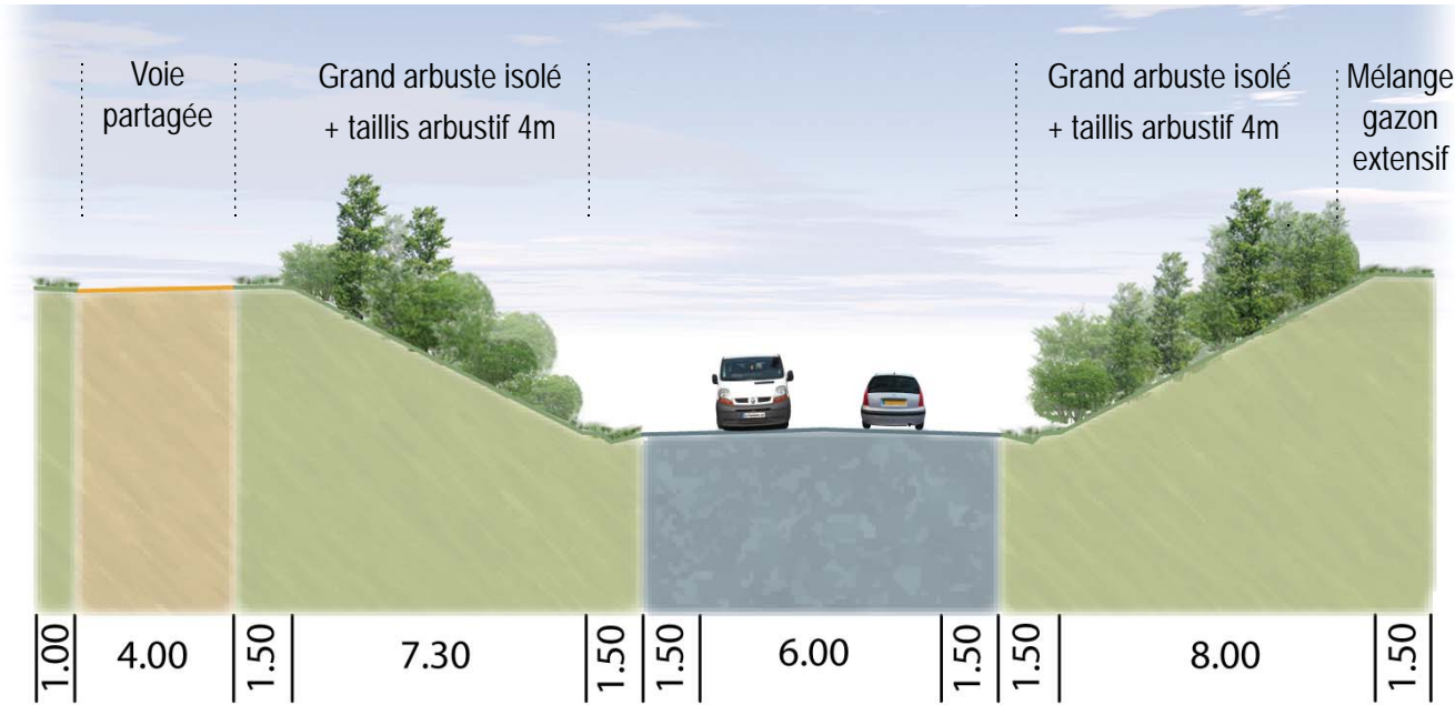
COUPE A-B PERCEPTION DE L'AUTOMOBILISTE UNE AMBIANCE CHAMPÊTRE ET RYTHMÉE EN LIEN AVEC L'ENTRÉE DE VILLE Profils 1 à 22
